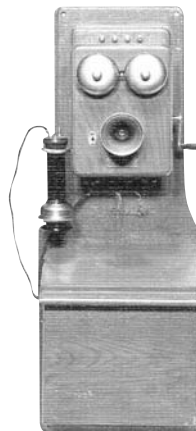
1896年デルビル磁石式電話機
